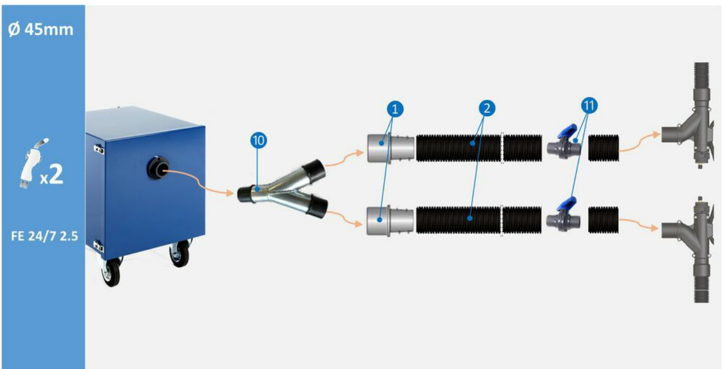
Tilbehørskonfiguration til to brugere, 45 mm tilslutning til svejseapparat. (10) Forgøring 50/50/50, art.nr. 55999420 (1) Slangetilslutning M50-44P, art.nr. 55999418 (2) Slange Superflex Ø 45 mm, sort 5 m, art.nr. 55999411 (11) Kugleventil 44 mm, art.nr. 55999422
